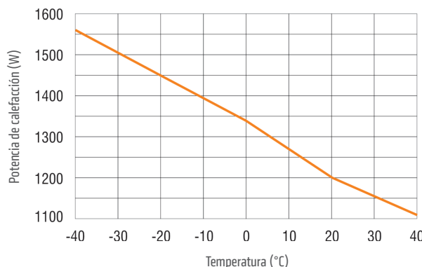
Diagrama de capacidad calorífica/temperatura ambiente CS 030
